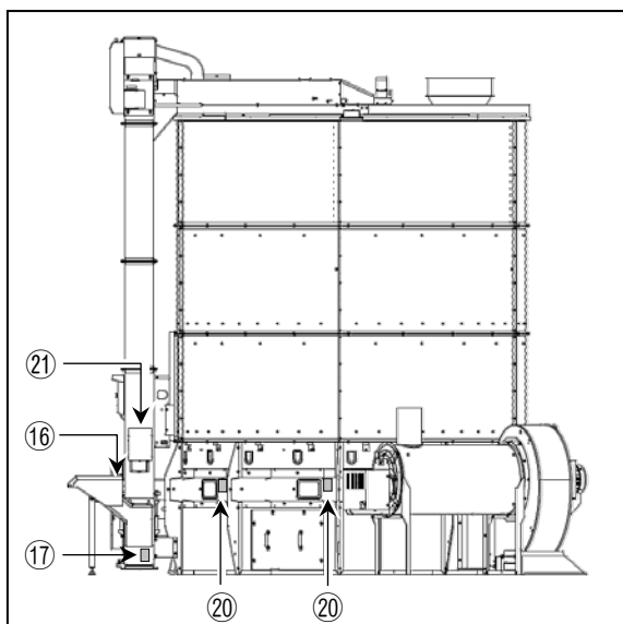
(右側面)
