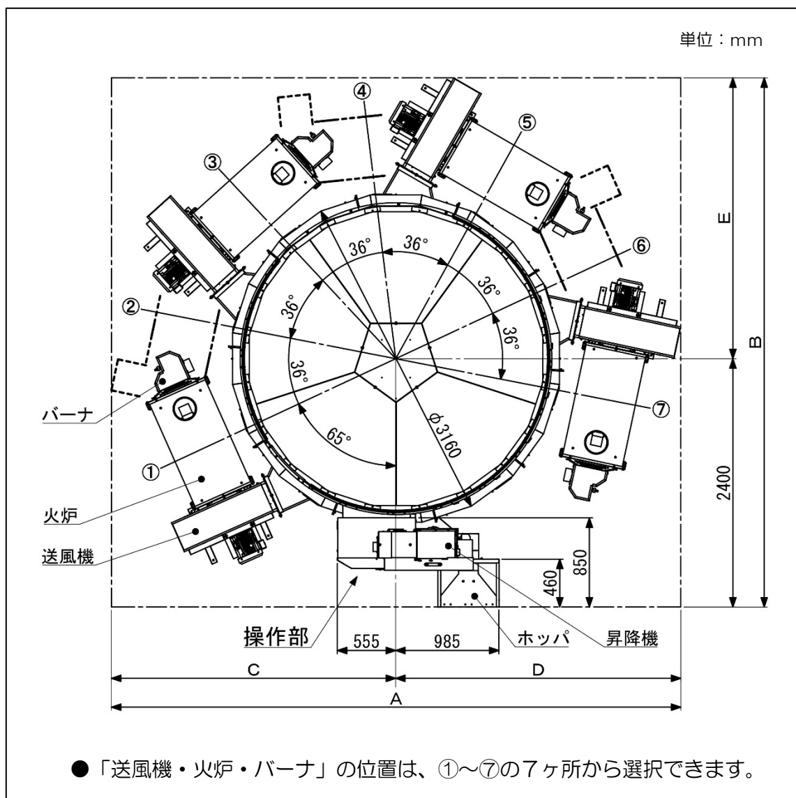
●「送風機・火炉・バーナ」位置による設置平面の寸法
