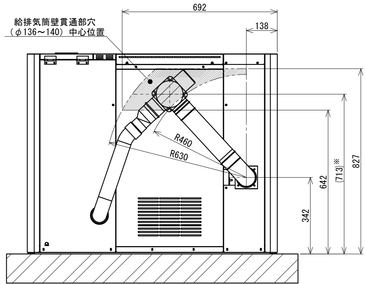
A-A 断面図
