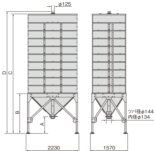
ベルトコンベヤ用(単位：mm)
